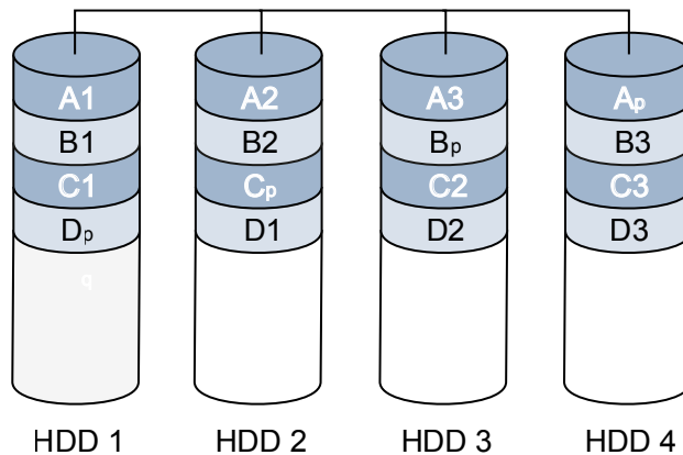
Abb. 9 RAID5 mit verteilten Daten (z.B. A1 bis A3) und Paritäts-Daten (z.B. Ap)
