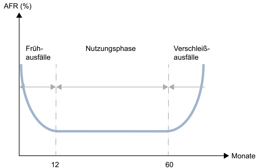
Abb. 4 Badewannenkurve (theoretisches Modell)
