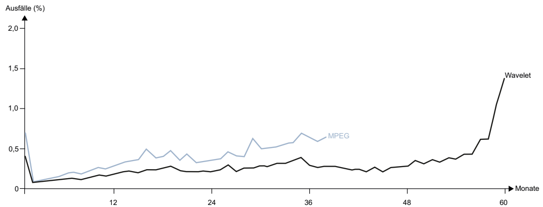
Abb. 6 Festplattenausfälle Anfang 2000 bis Ende 2005
