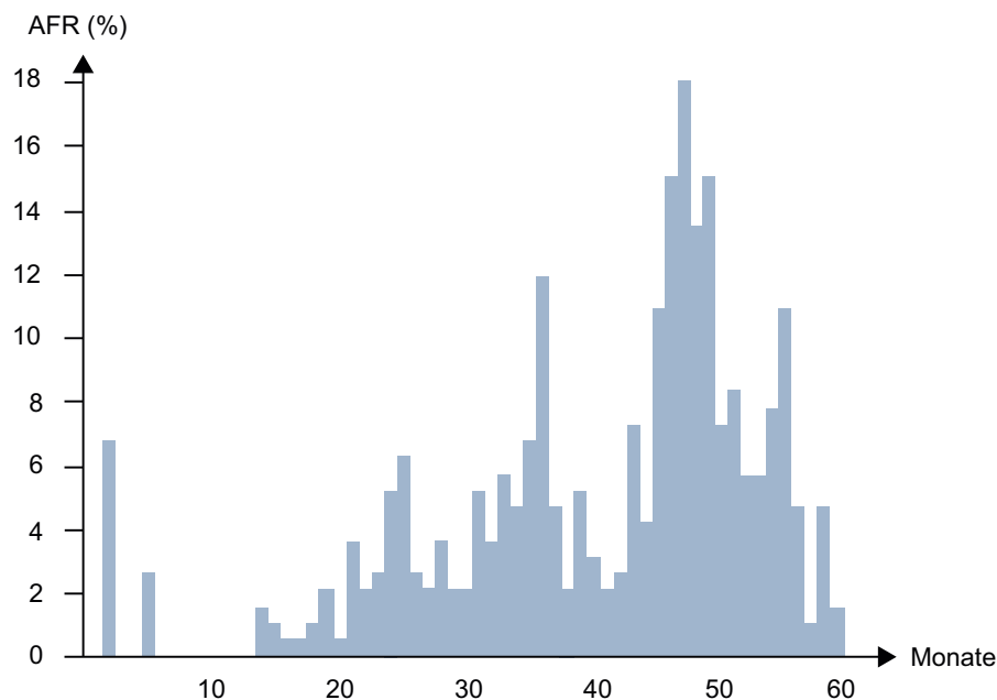
Abb. 5 Ausfallverteilung
