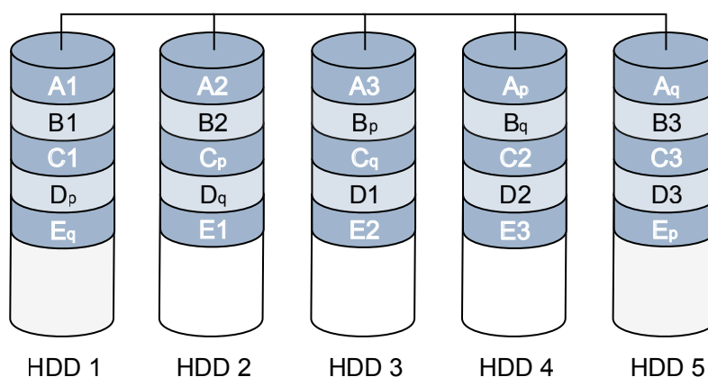
Abb. 10 RAID6 mit verteilten Daten (z.B. A1 bis A3) und doppelten Paritäts-Daten (z.B. 2 \times A_p )
